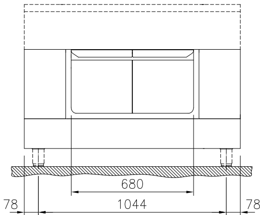
Zij aanzicht
